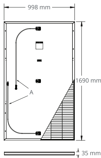
Perfil de bastidor
